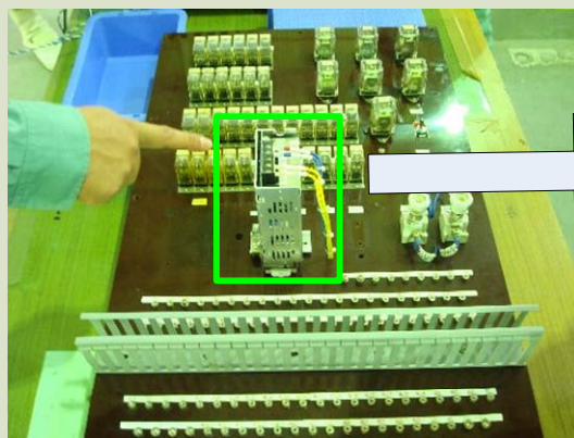
電源装置(新品)取り付け状況
