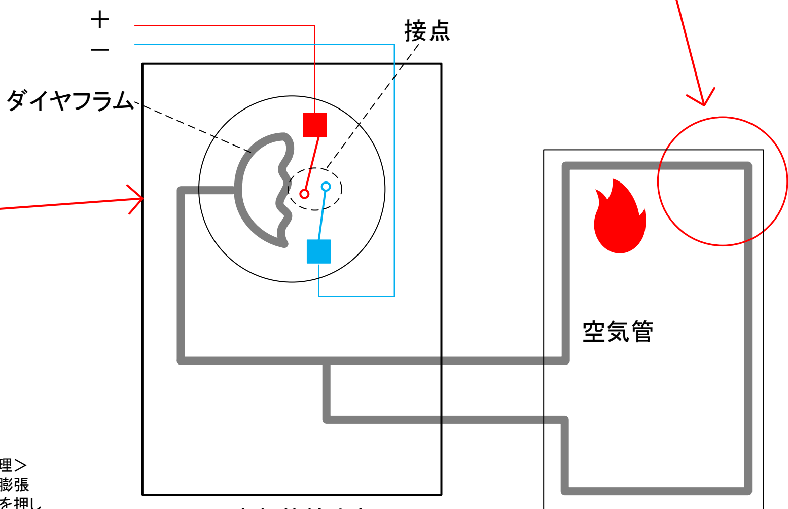
空気管検出部
