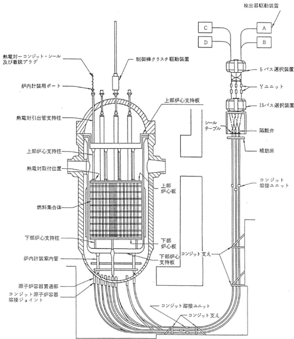
炉内核計装装置概要図
